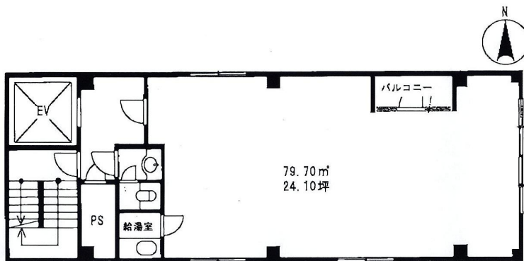
○2F～4F平面図
